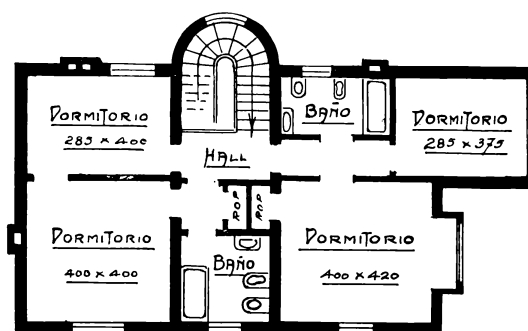
— PLANTA ALTA —
