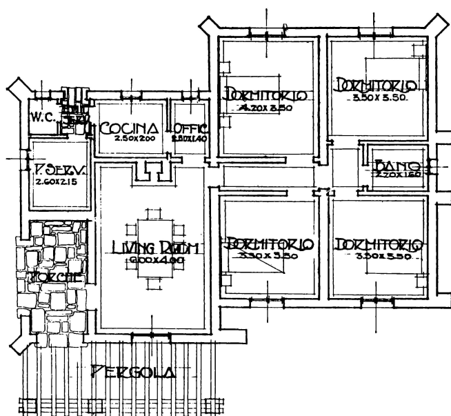
PLANO DE LA CASA TIPO D
