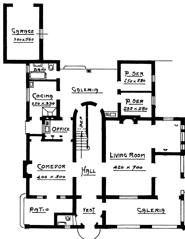
— PLANTA BAJA —
