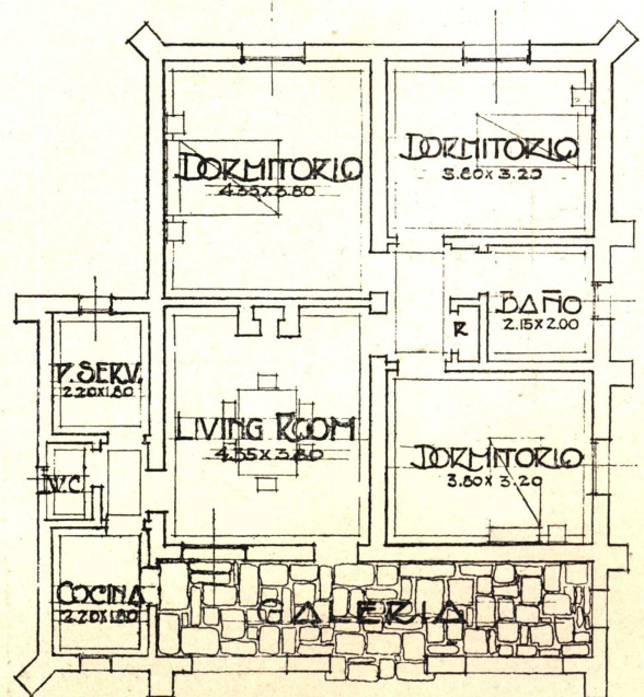
PLANO DE LA CASA TIPO C
