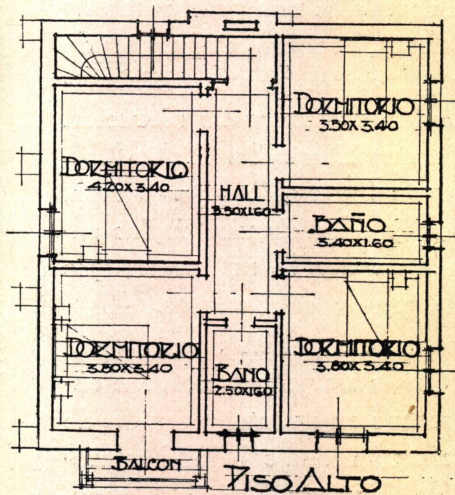
PLANOS DE LA CASA TIPO E
