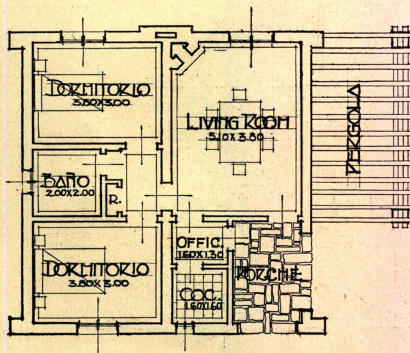
PLANO DE LA CASA TIPO B
