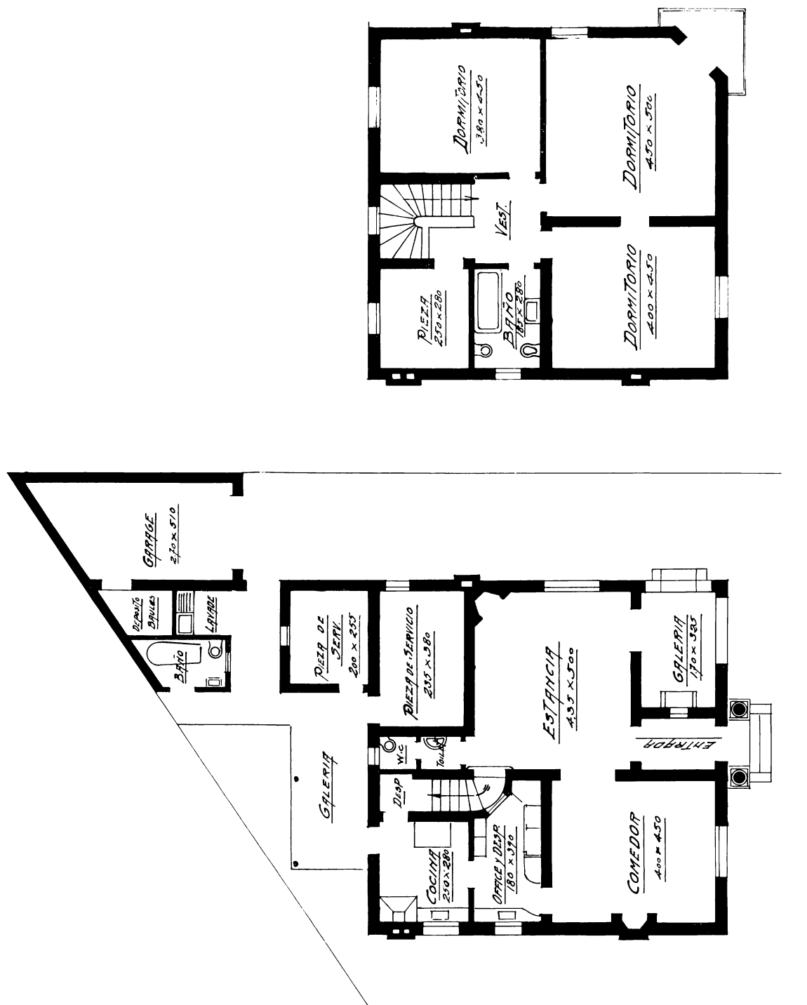
PLANTA BAJA
