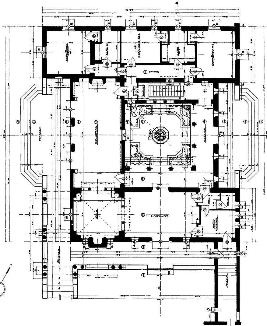
PLANTA BAJA Escala 1:50.00
