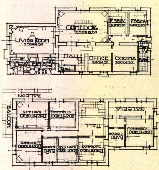
PLANOS DE LA CASA TIPO F
