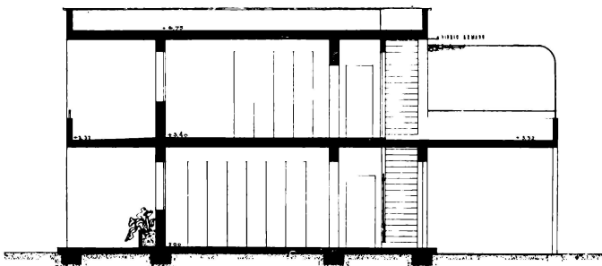
CORTE A-B ESCALA 1:200
