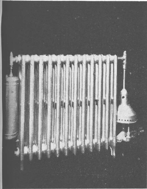
40, Estufa eléctrica de reflexión con carga de 2 kwh. Fimexa, S. R. L. 41, Radiador hidrotérmico eléctrico "Neograf" a termosifón, modelos de 7, 10, 12, 14, 16 y 20 secciones. Pablo Rocco e Hijo, S. R. L. 42, Radiadores eléctricos "Isothermos". De 8, 13 y 20 elementos para ambientes de 40, 65 y 110 metros 3 y consumos de 1200, 1500 y 2500 watts. Copimex Com. e Ind. 43, Radiador hidrotérmico "Neograf" a gas con los mismos números de elementos del número 41. Pablo Rocco e Hijo, S.R.L. 44, Caloventilador que produce calor en invierno y frescura en verano. Para corriente alternada 220, en colores variados. Establecimientos E.M.E.T.A. S. R. L. 45, Estufa eléctrica "Kalorik" en distintos colores y modelos A. C. E. C. Argentina.
