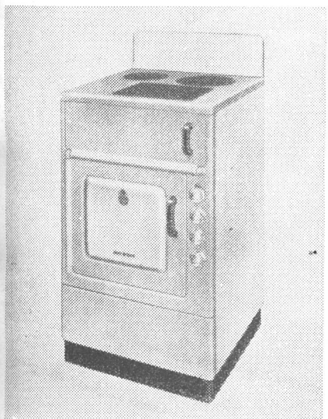
51 , Cocina a gas "Vesta" de dos hornallas y horno. Dimensiones exteriores: 0,82 de alto, 0,53 de ancho (en la plancha) y 0,47 de profundidad. Quemadores desmontables en hierro fundido y distribuidor de llama en bronce. M. Drutman é Hijos. 52 , Cocina a gas "Kowa" modelo Mendoza, con cuatro quemadores comunes, uno doble concéntrico, dos hornos y grill. Dimensiones: 1,17 de ancho, 0,60 de profundidad y 0,81 de alto. Quemadores de aluminio, plancha superior a bisagras. Ricardo Fritzsche. 53 , Cocina de lujo de cuatro quemadores con prusiana. Tipo especial para casas de familia. Malugani Hnos. 54 , Cocina eléctrica terminada en crema y verde. Fimexa S. R. L. 55 , Cocina a gas de tres quemadores, con horno amplio. Malugani Hnos. 56 , Cocinas a gas "Laurens" de tres quemadores. Medidas: 0,86 de altura, 0,60 de frente, 0,53 de profundidad. Talleres Angel Ottolenghi.
